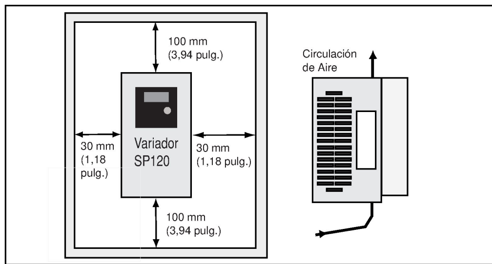
Figura 2.1 – Espacios libres mínimos de flujo de aire
