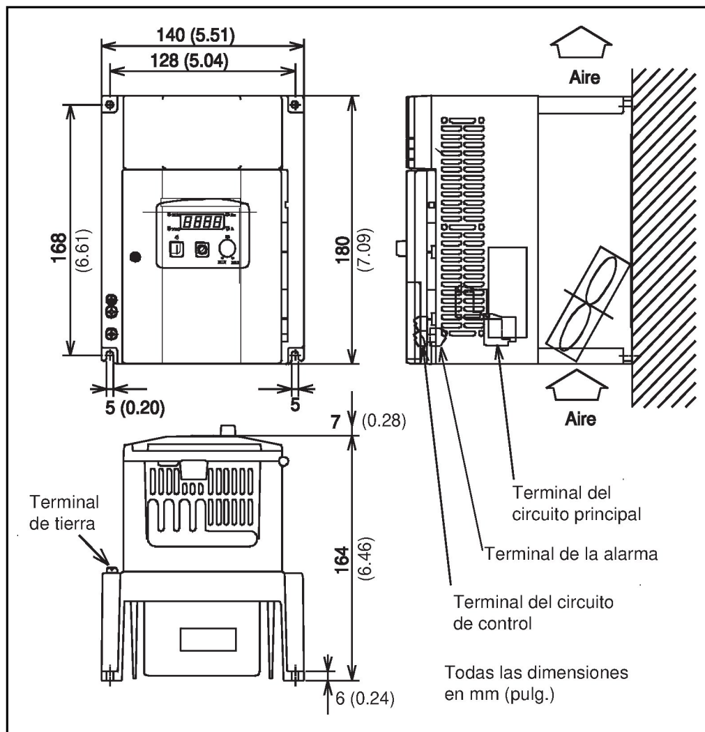
Figura A.4 – Dimensiones del S12-20010/20015/408P6
